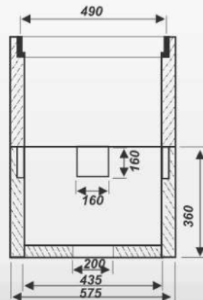
Przekrój poprzeczny
