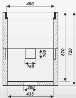
Przekrój podłużny
